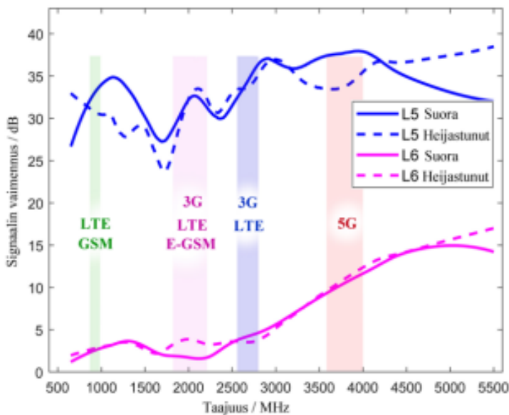
Kaksilasisten lasipakettien L5 ja L6 vertailu, suora ja heijastunut signaali
